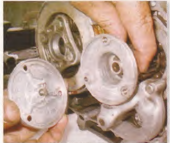
Interior del filtro centrífugo de aceite
